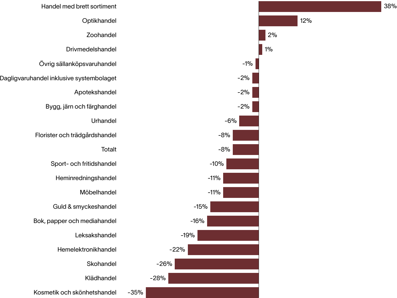
Fig. 13. Källa: Butiksdatan
